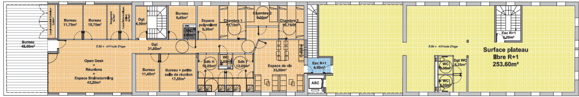
PLAN NIVEAU R+1
