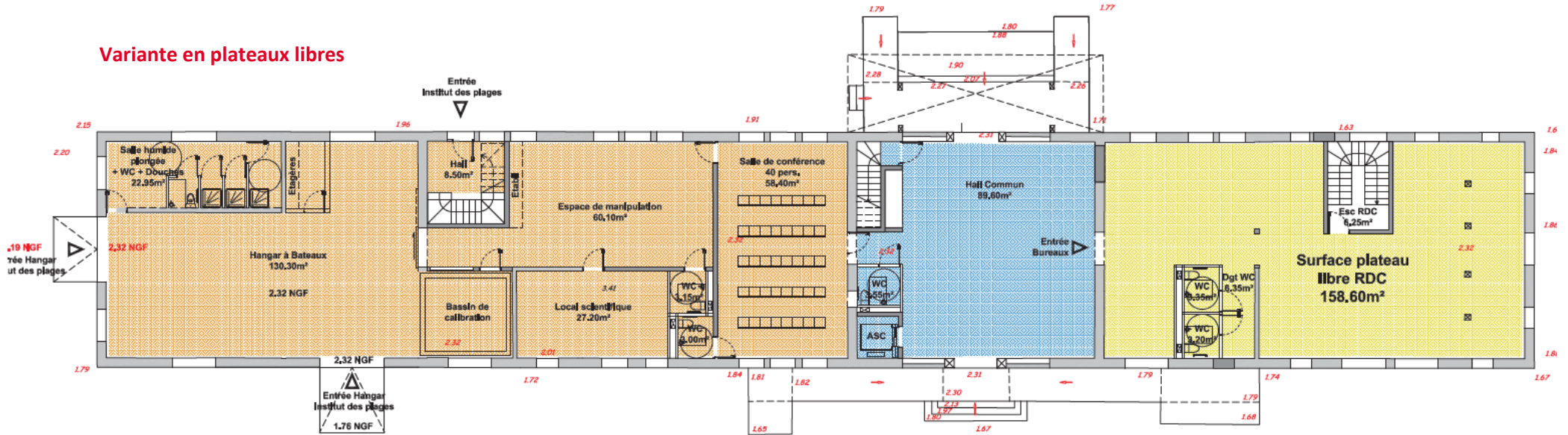
PLAN NIVEAU RDC
